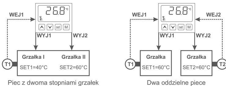
Piec z dwoma stopniami grzałek
